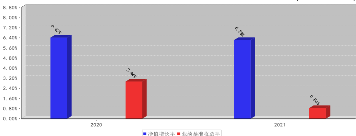
浙商智多兴稳健一年持有期C基金每年净值增长率与同期业绩比较基准收益率的对比图(2021年12月31日)
