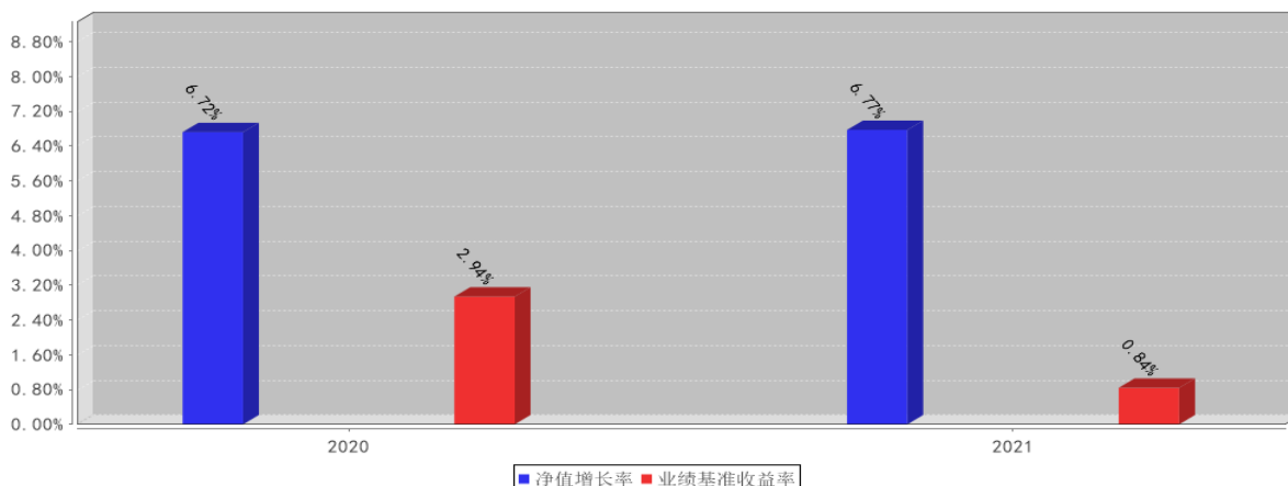
浙商智多兴稳健一年持有期A基金每年净值增长率与同期业绩比较基准收益率的对比图(2021年12月31日)
